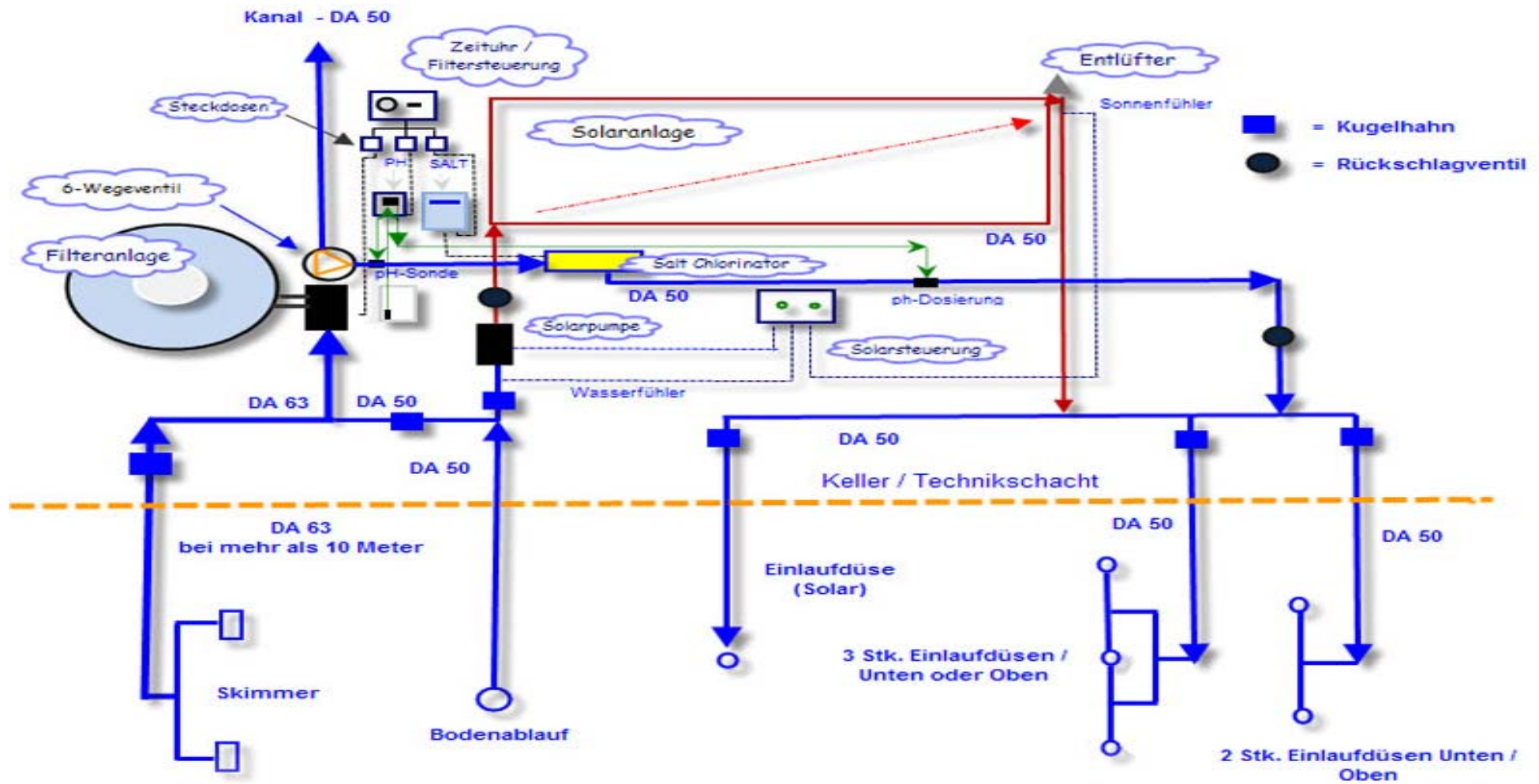
Installationschema:
