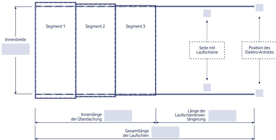
Grundriss der Überdachung (Masse in cm)
