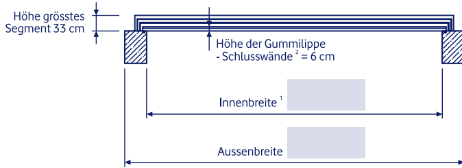
Frontansicht der Überdachung (Masse in cm)
