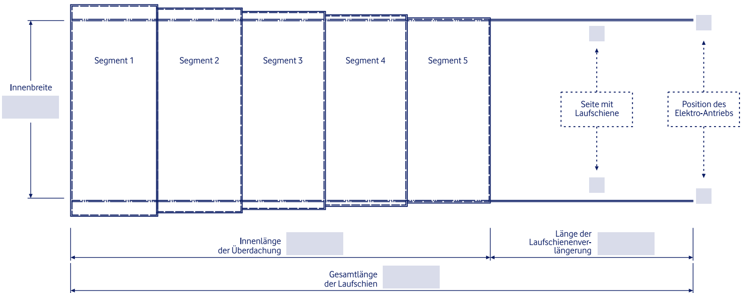
Grundriss der Überdachung (Masse in cm)
