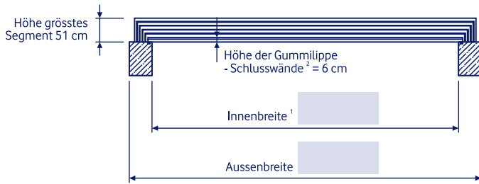
Frontansicht der Überdachung (Masse in cm)
