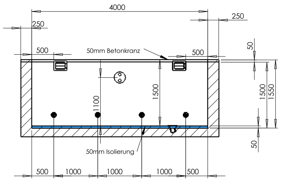
SCHNITT A-A
