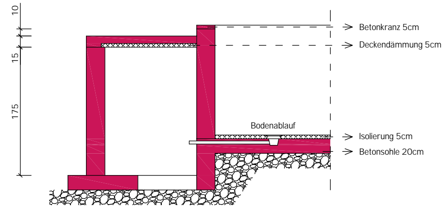
Schachtabsenkung um 50cm
