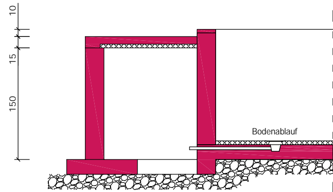
Schachtabsenkung um 25cm
